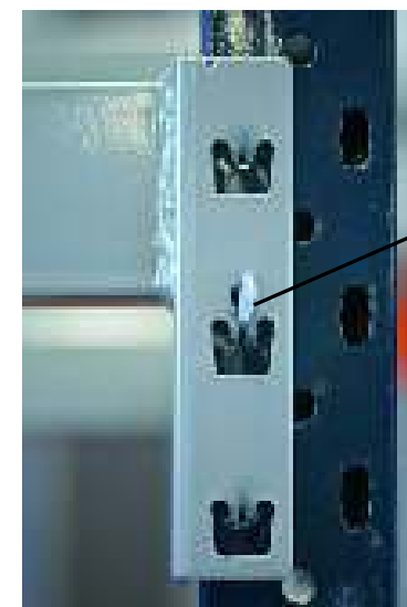
Sikkerhedsbøjler til sikker fastholdelse af hyldebjælker
